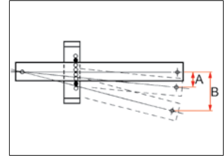
شکل ۲۳: حالت انحرافی مالبند از سوراخ وسط
