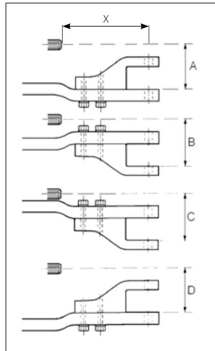
شکل ۲۱: تنظیم ارتفاع مالبند
