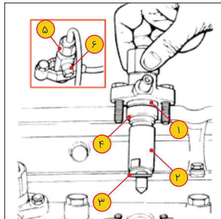
شکل ۲۸: تعویض انژکتور
